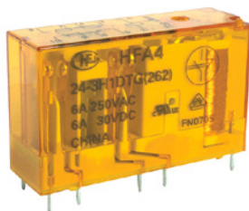
relé HFA4
