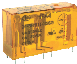
relé HFA4
