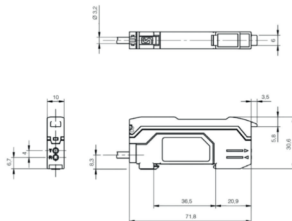
Rozměry (mm)
