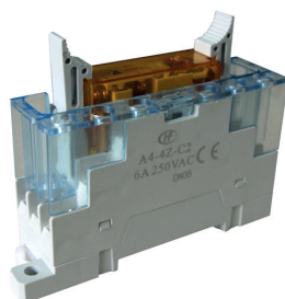
patice A4-4Z-C2
