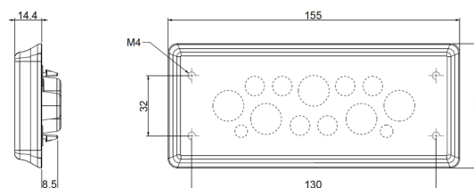
Rozměry (mm)
