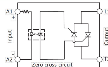
Zapojení:
