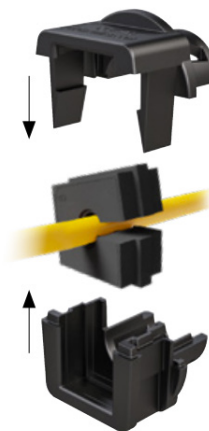
Montáž vložky do průchodky
