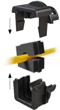
Montáž vložky do průchodky
